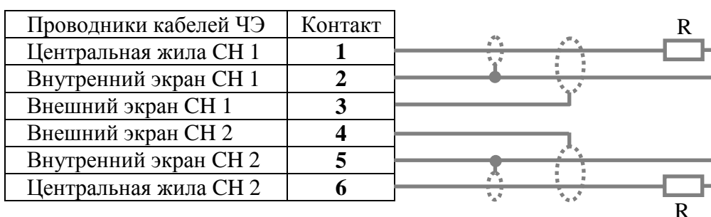
Рис. 8.2. Электрическая схема подключения кабелей чувствительных элементов
