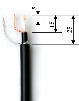
Рис. 8.3. Образец разделки кабелей ЧЭ для подключения к БОС
